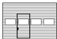
Plná ocelová vrata s prosklením a integrovanými personálními dveřmi
